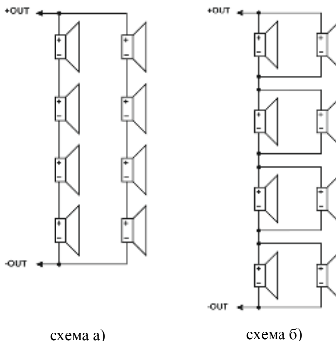
Рис. 9 Вариант 3 подключения РО
