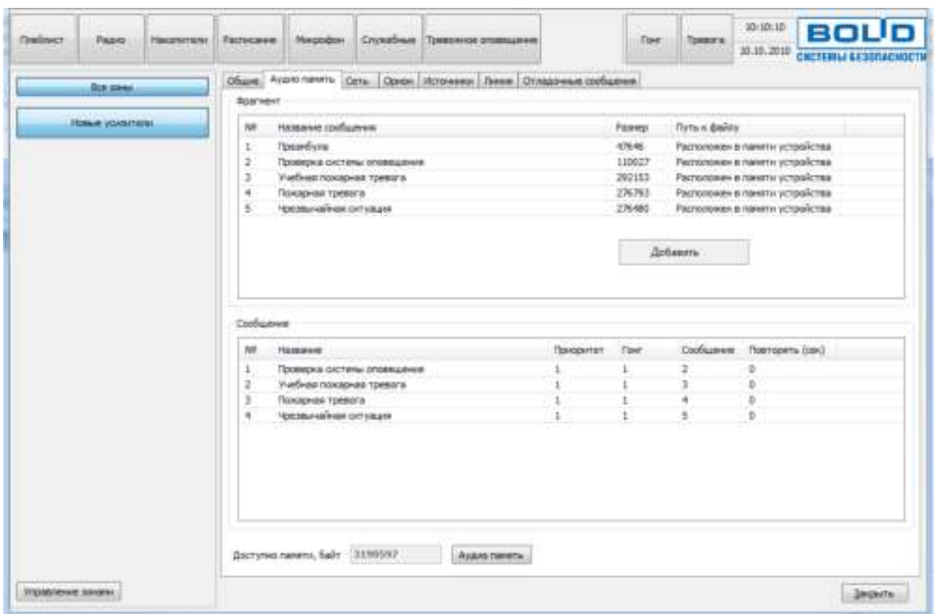
Рисунок 2.2.8. Свойства памяти блока
