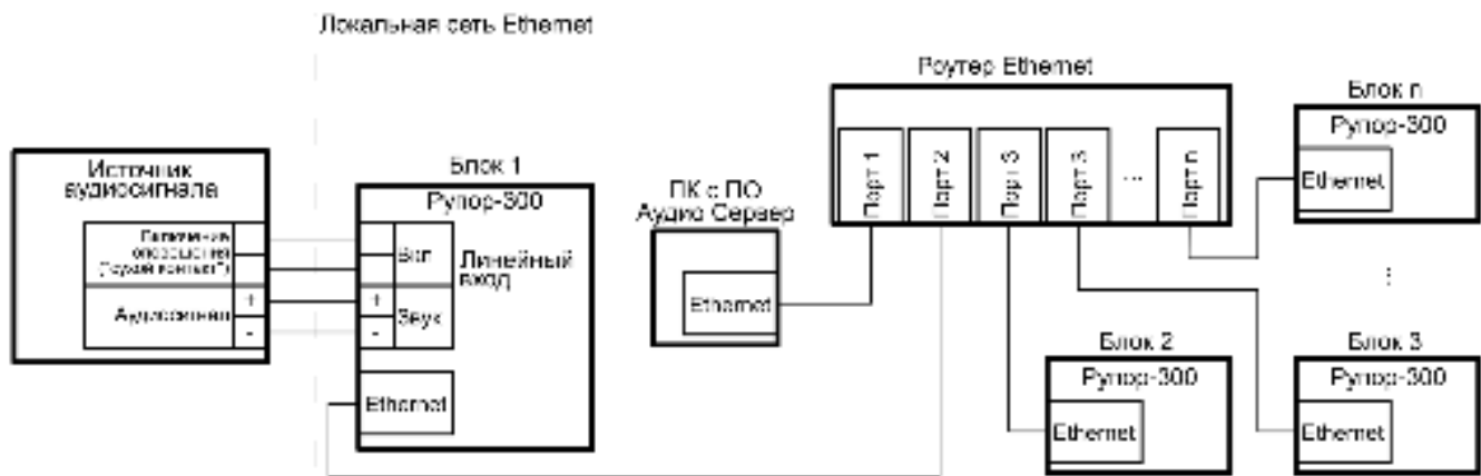
Рисунок 2.2.4. Схема организации сети с одним источником звукового сигнала.
