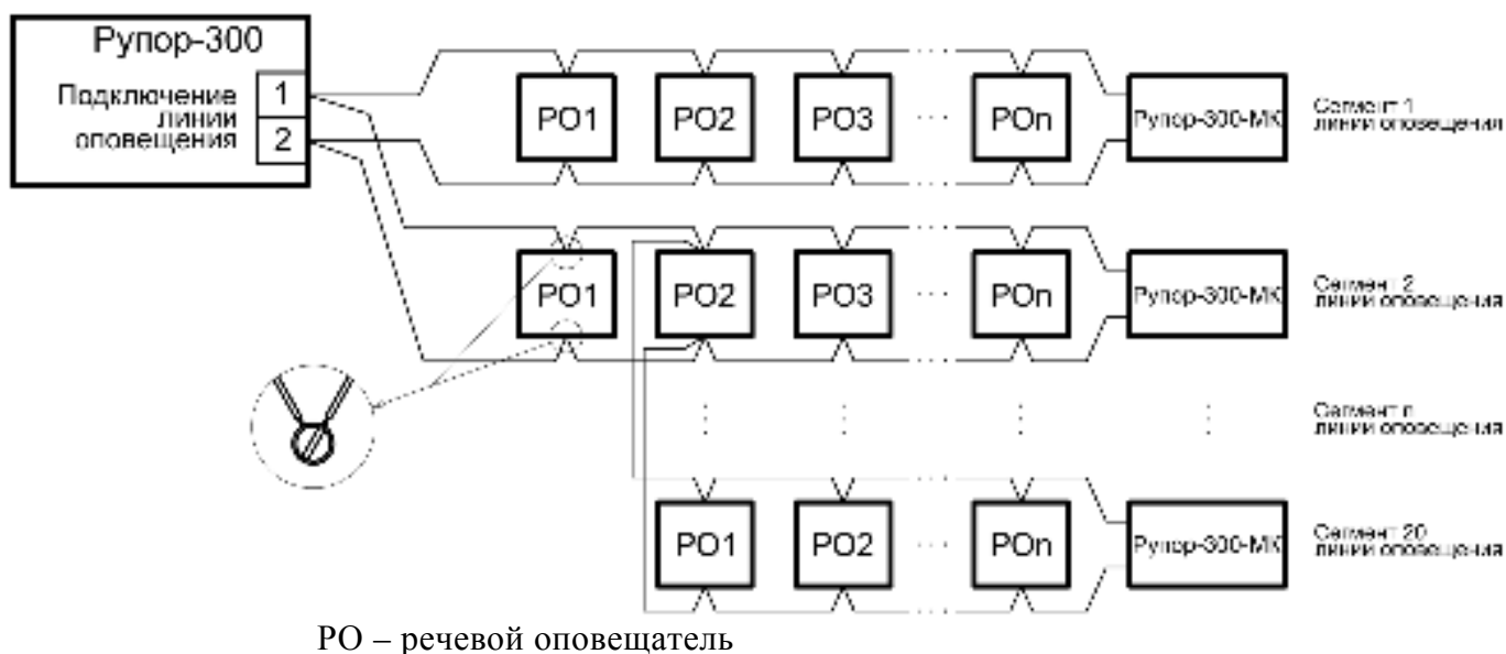
Рисунок 2.2.5. Подключение громкоговорителей к линиям оповещения
