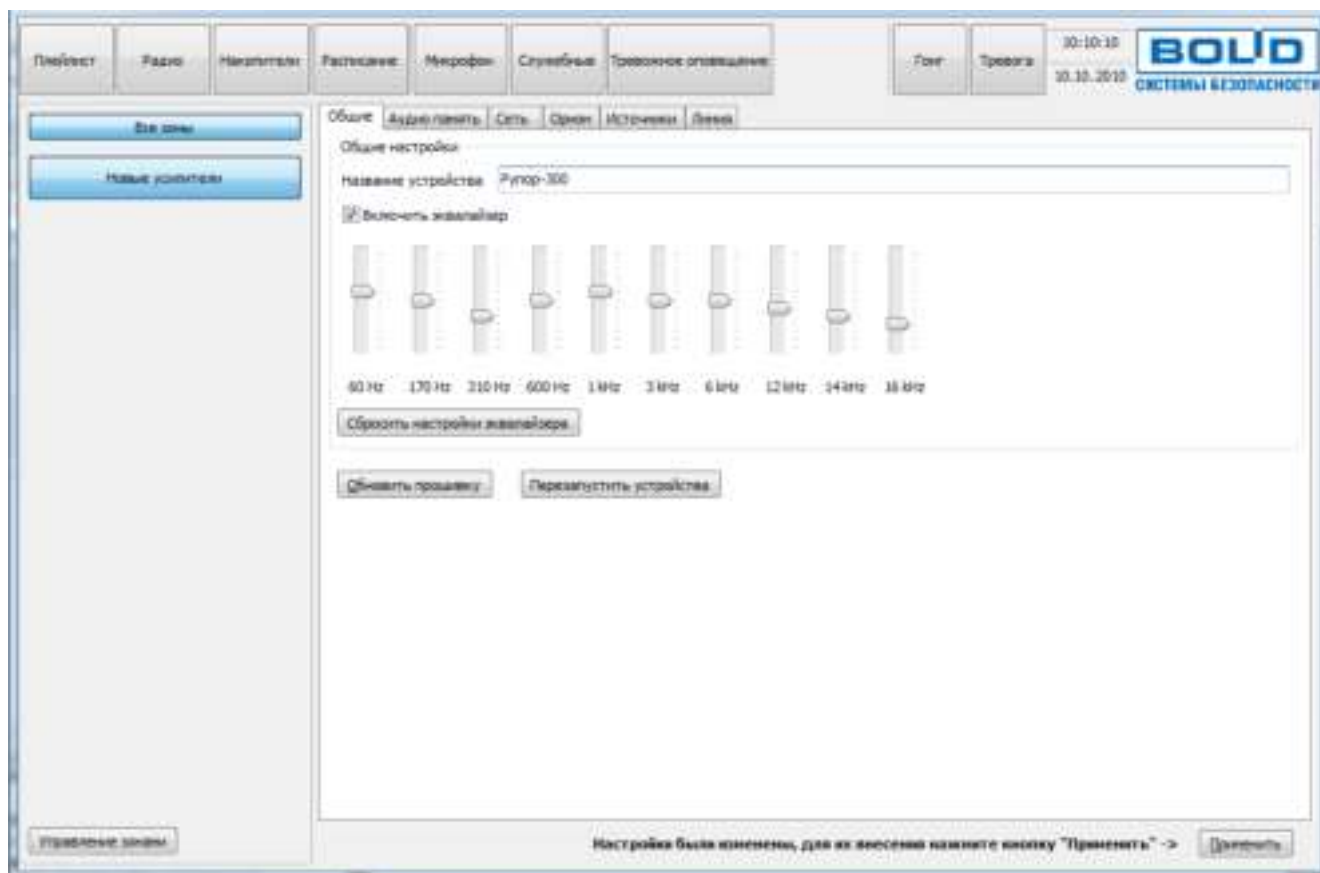
Рисунок 2.2.7. Окно конфигурирования блока
