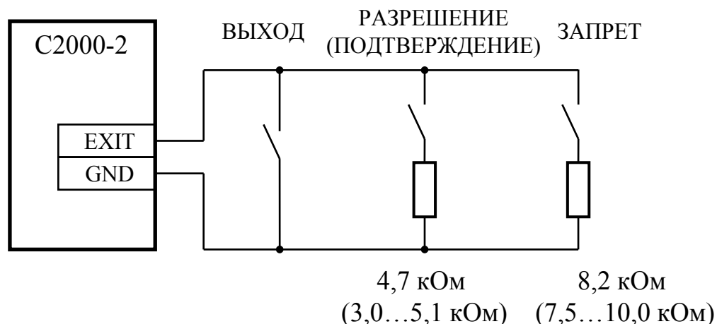
Рисунок 5 Схема подключения кнопок "ВЫХОД", "РАЗРЕШЕНИЕ" и "ЗАПРЕТ"
