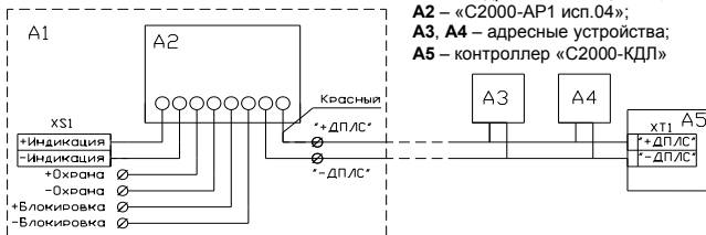
Рисунок 1 Схема соединений
