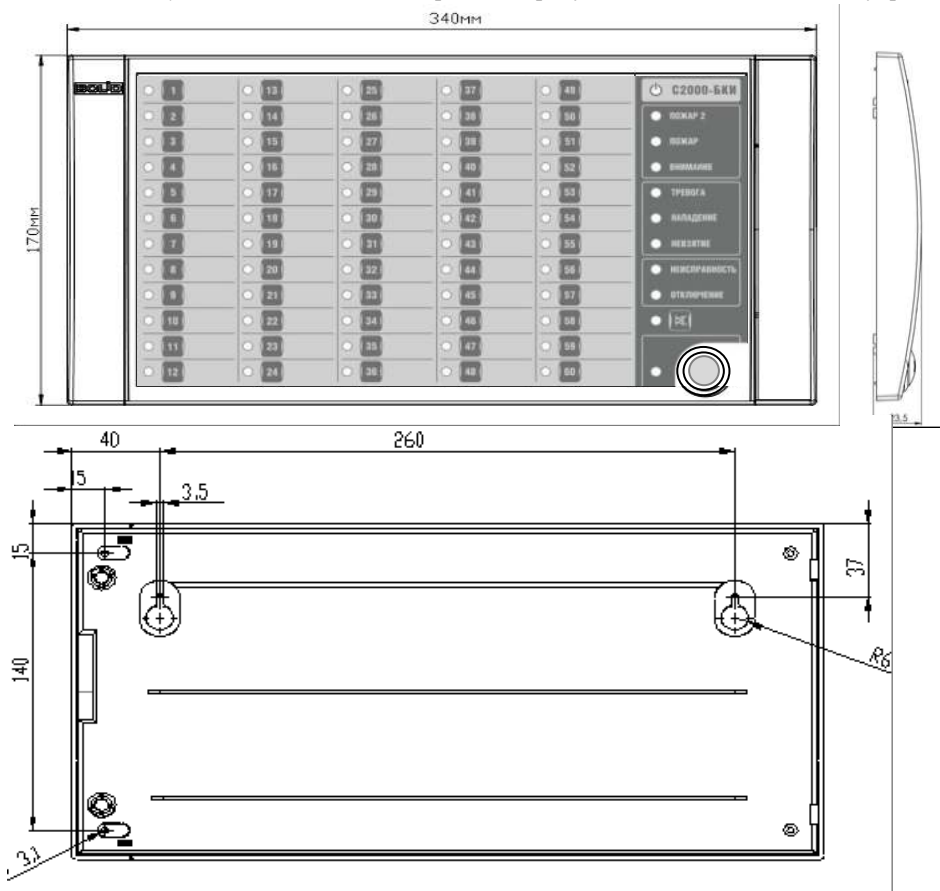
Рисунок 1. Внешний вид, габаритные и установочные размеры блока
