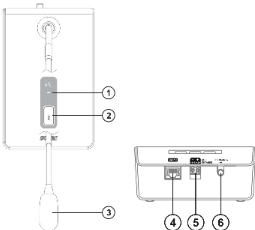
Рисунок 1 - Лицевая и задняя панели пульта
