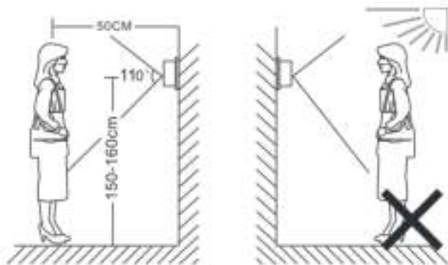
Рис. 3 Рекомендуемое расположение для монтажа
