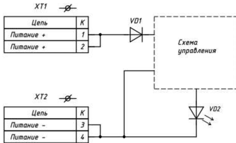
Принципиальная схема извещателя ИПР 535 Горизонт
