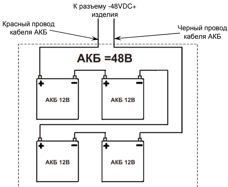
Рисунок 5 — Схема монтажа аккумуляторной батареи.
