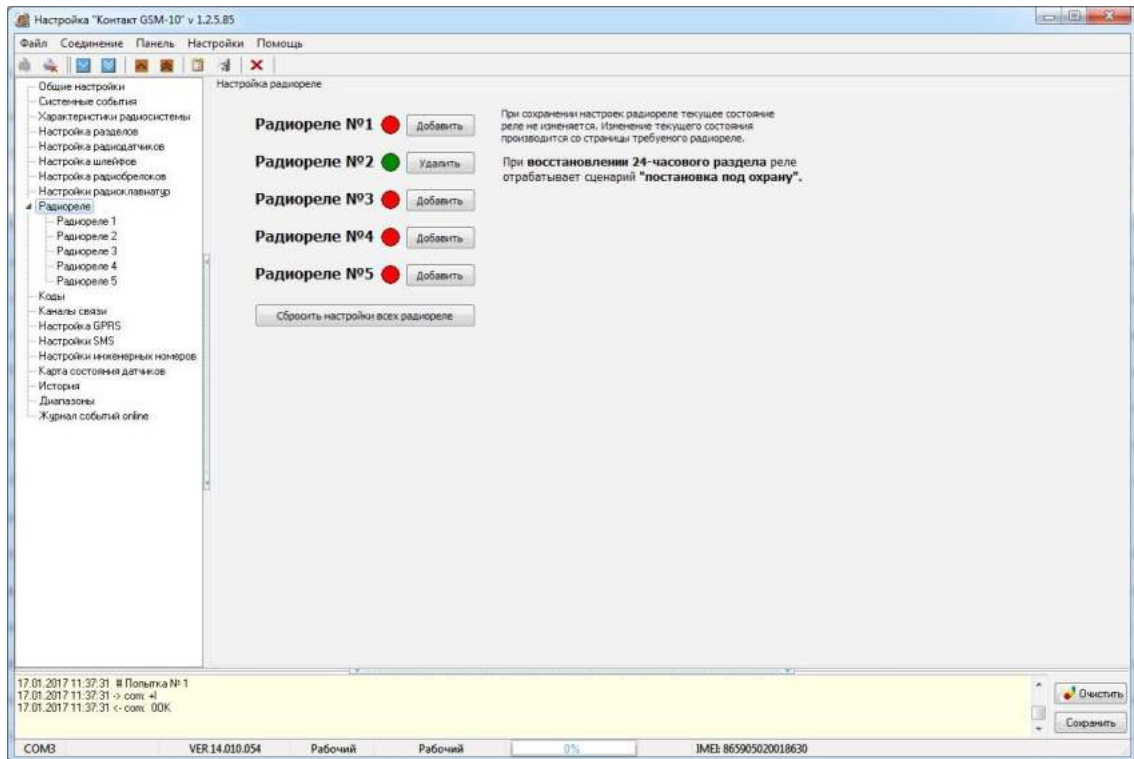
Рисунок 24. Раздел «Радиореле»
