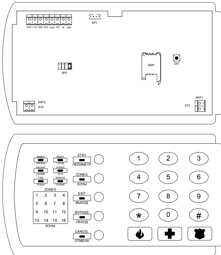
Рисунок 2. Контакт GSM-10
