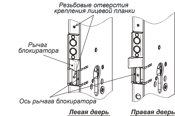
Рис. 4. Положение блокиратора на левой и правой двери
