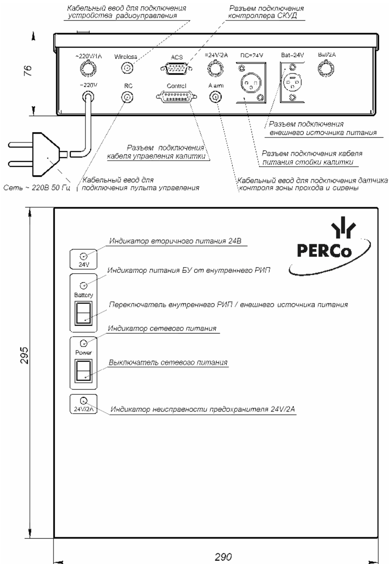
Рисунок 5. Блок управления
