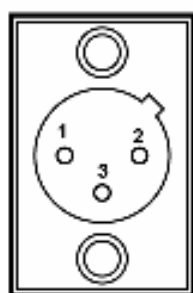
Рисунок 6. Назначение контактов разъемов БУ
