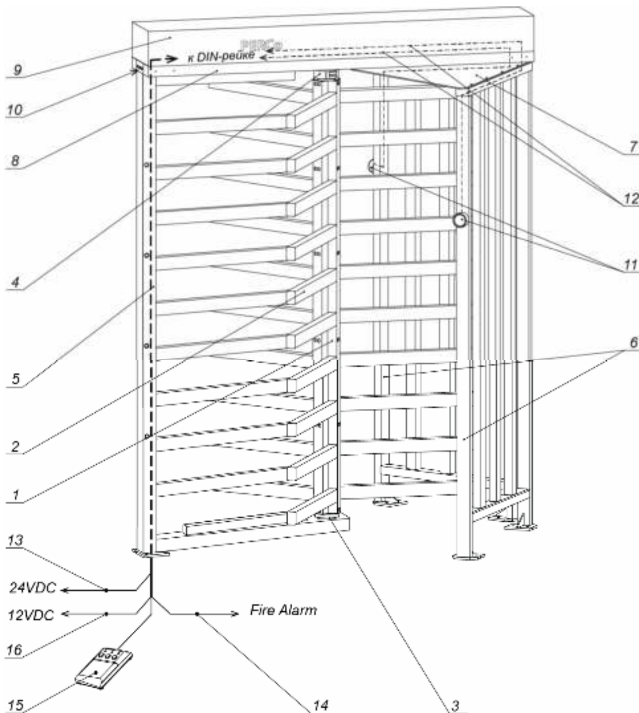
Рисунок 2. Устройство турникета
