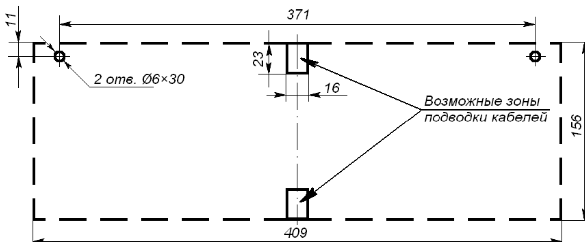
Рисунок 4. Схема разметки для установки ТСВ (пунктиром показаны габариты изделия)
