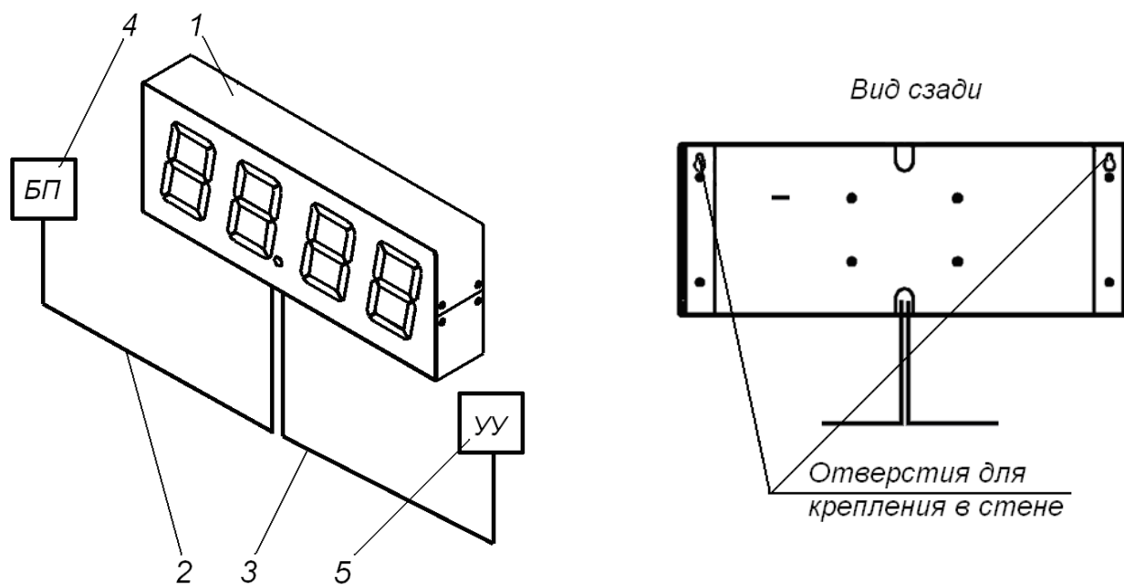
Рисунок 1. Устройство ТСВ:
