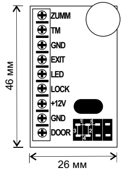
Рис.2 Внешний вид платы
