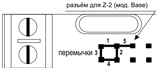
Рис. 3 Положение перемычек
