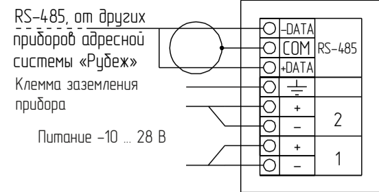
Рисунок 2 – Схема подключения прибора
