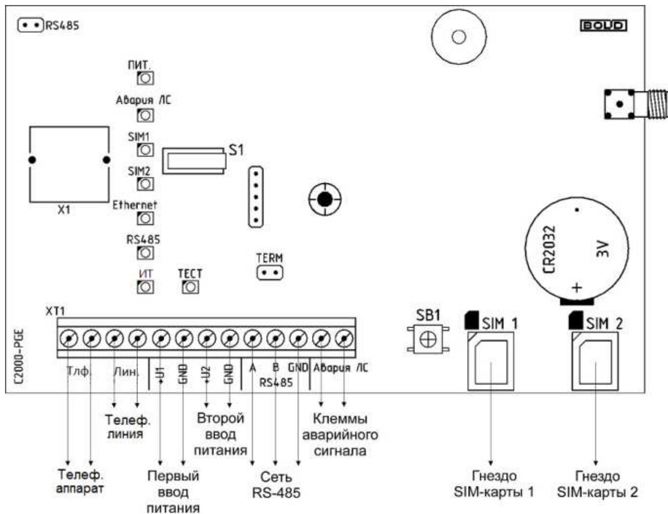
Рисунок 8.4 Схема подключений «C2000-PGE»
