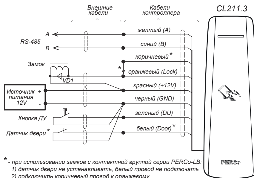
Схема подключения контроллера PERCo-CL211.3.
