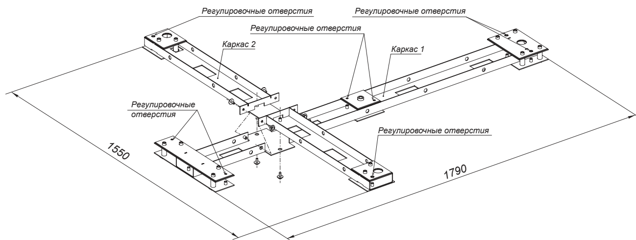
Установка рамы
