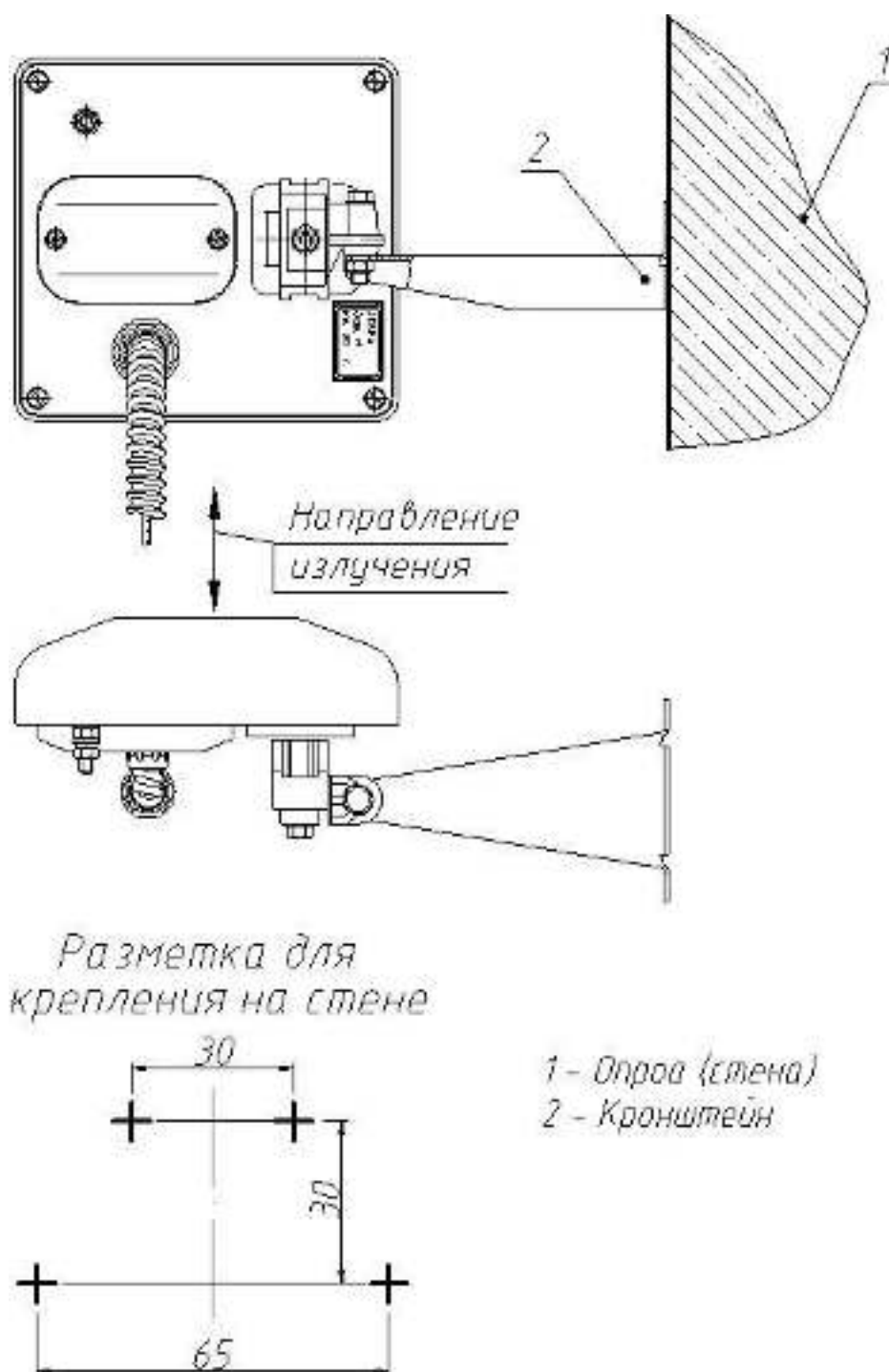
Рисунок 6.3 Установка извещателя на стене с использованием «Кронштейна-120» (варианты исполнения – все)
