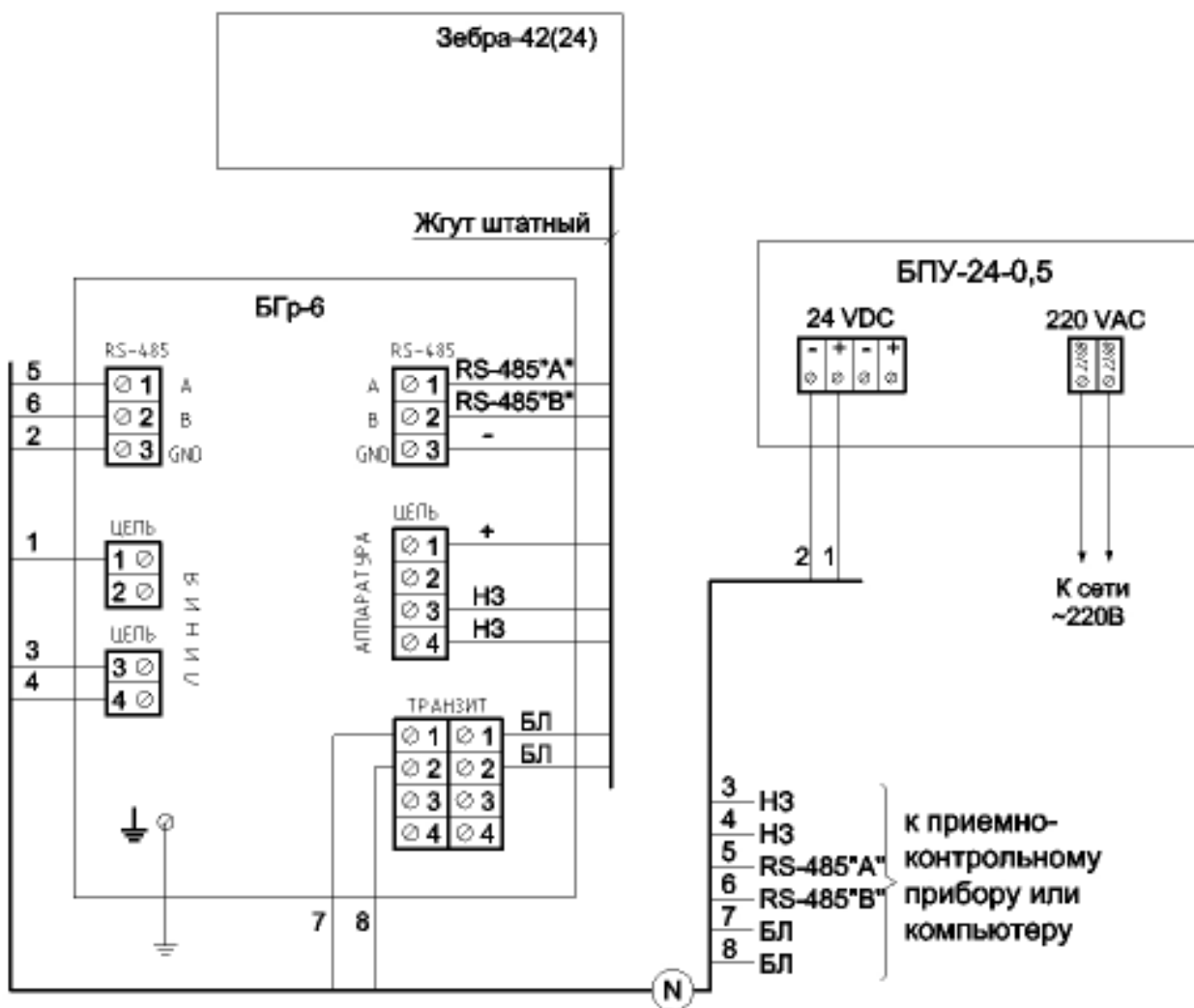
Рисунок - 2.8 Схема подключения извещателя при использовании блока грозозащиты «БГр-6».
