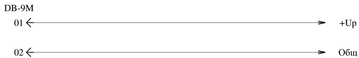
Рисунок 1.2 - Схема электрическая принципиальная жгута Ж2
