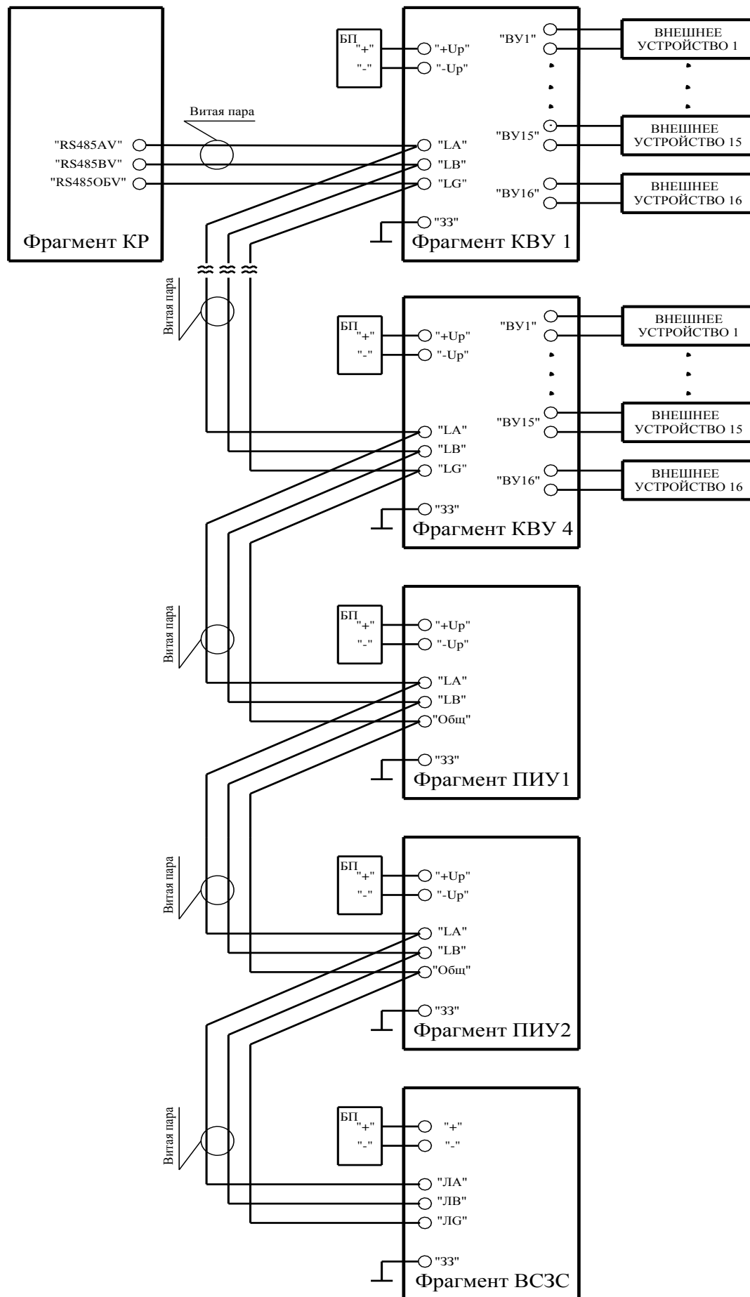
Рисунок 2.10 - Схема подключения КБУ-08, ПИУ, ВСЗС к КР
