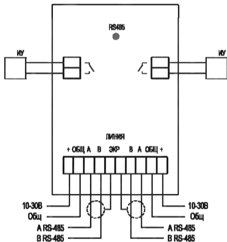
Рисунок 1 – Схема подключения
