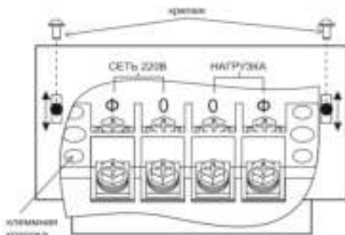
Рисунок 3 – Схема подключения к клеммной колодке
