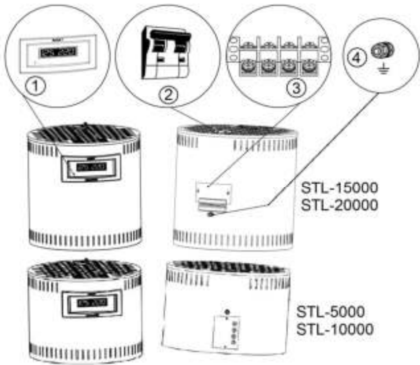
Рисунок 1 Общий вид стабилизатора и его функциональных элементов
