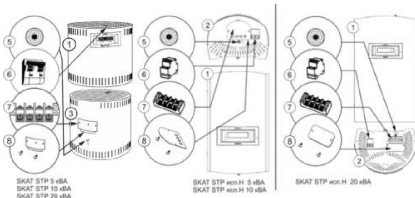
Рисунок 1. Общий вид стабилизатора и его функциональных элементов
