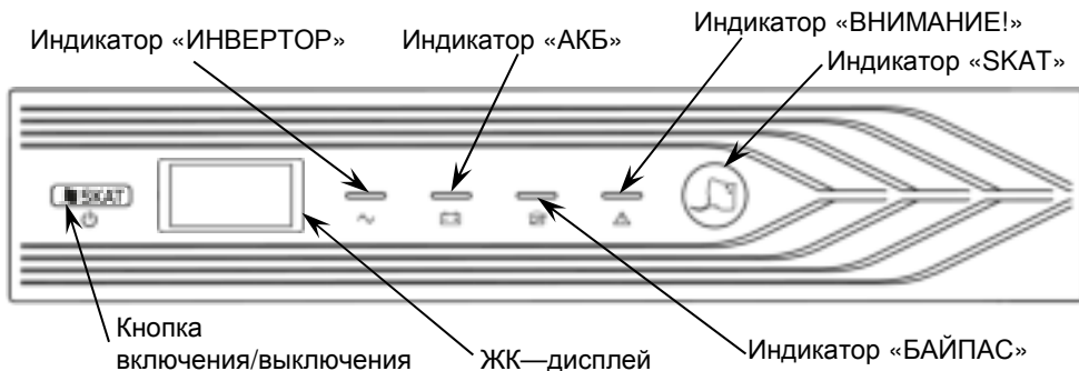
Рисунок 7 — Общий вид передней панели ИБП
