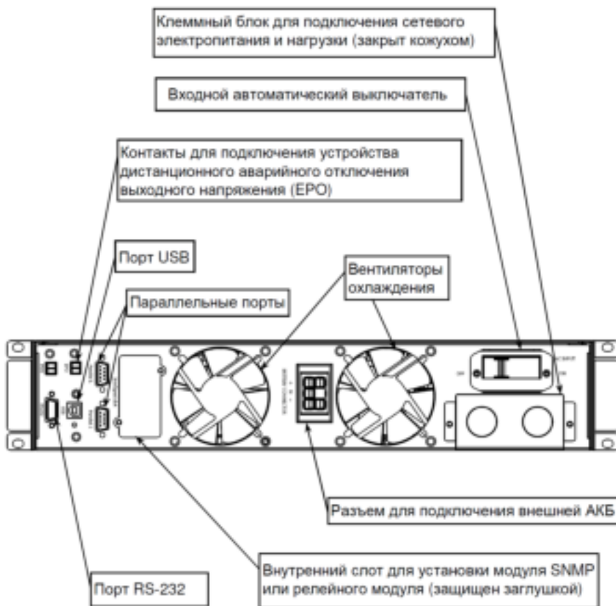
Рисунок 5 — Общий вид задней панели ИБП.
