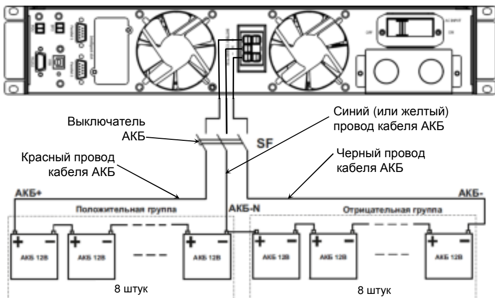
Рисунок 3 — Схема монтажа аккумуляторной батареи.
