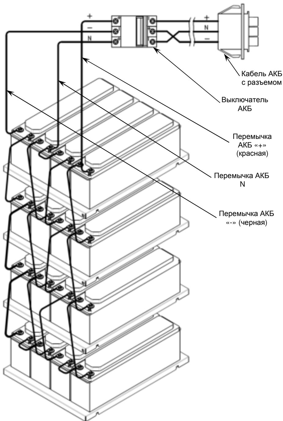
Рисунок 4 — Пример размещения и подключения на полках комплекса.
