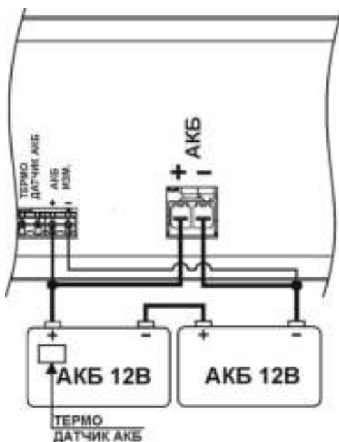
Рисунок 4 – Подключение АКБ и термодатчика АКБ.
