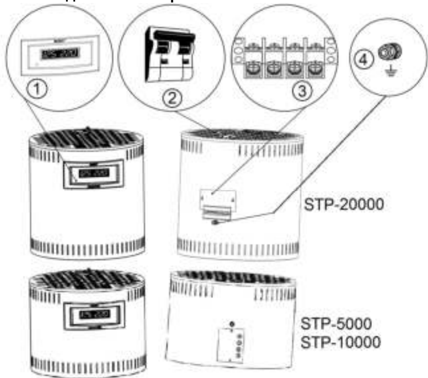
Рисунок 1 Общий вид стабилизатора и его функциональных элементов
