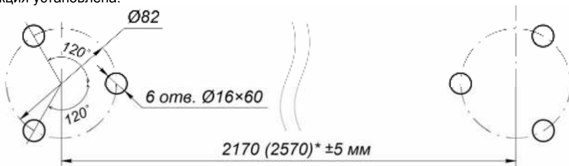
Рисунок 17. Схема разметки отверстий для установки фланцев двойной распашной секции ограждения с магнитным УБ
