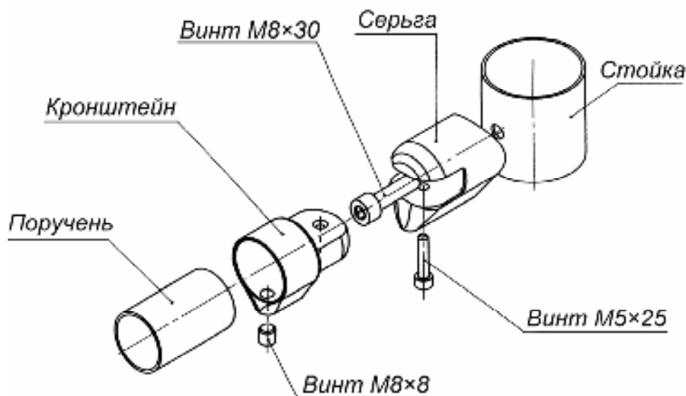
Рисунок 10. Схема крепления поручней к стойкам ограждения с использованием поворотного патрубка VN02 0-11
