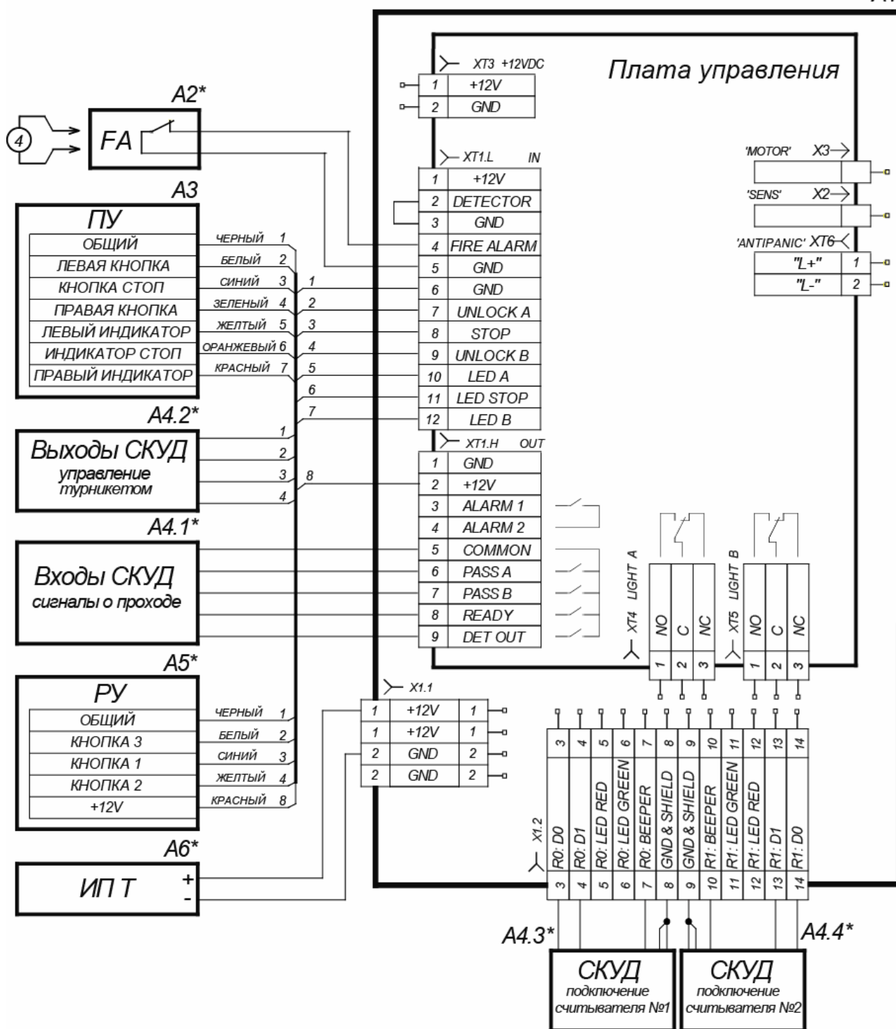
Рисунок 11. Схема соединений турникета и дополнительного оборудования 1
