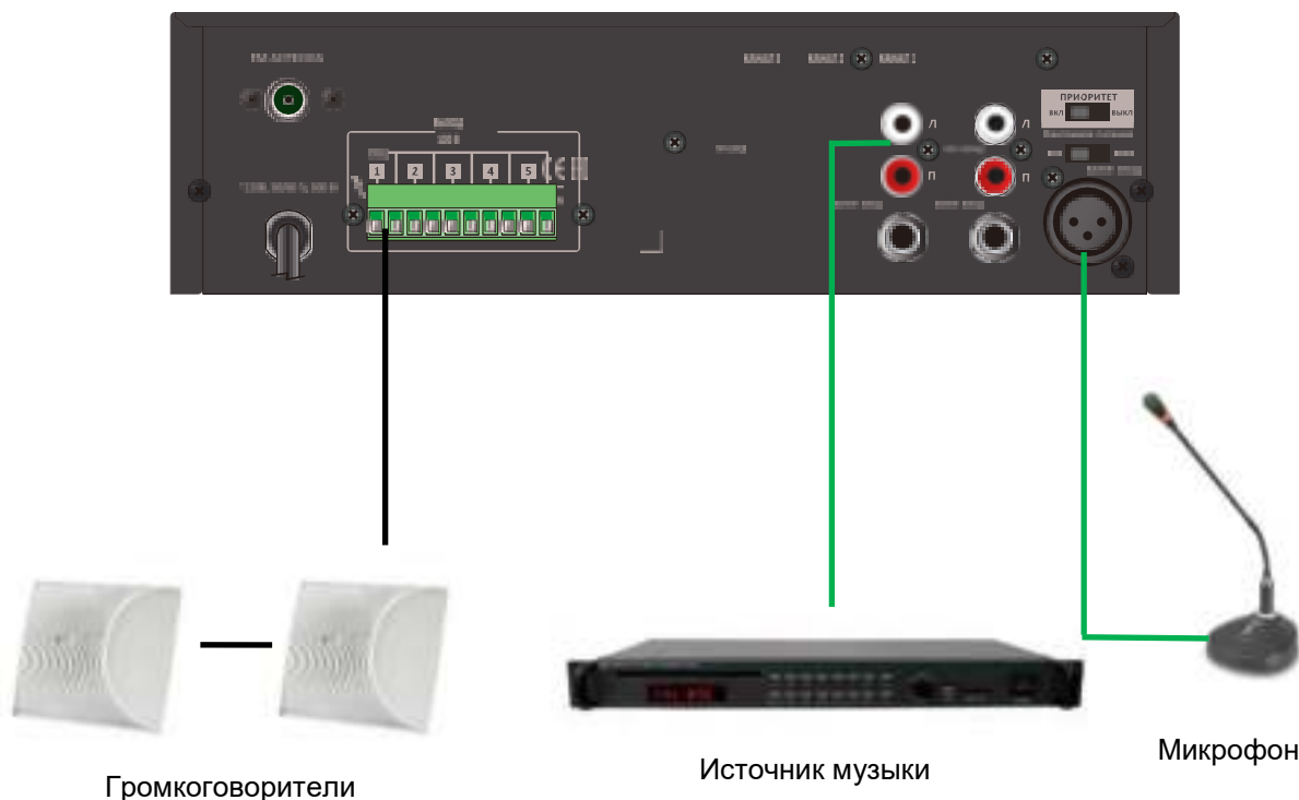
Рис. 2.1. Схема подключения LPA-TA-650MZ
