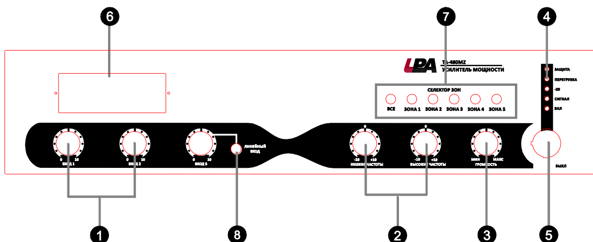
Рис. 3.1. Схема расположения средств управления LPA-TA-650MZ
