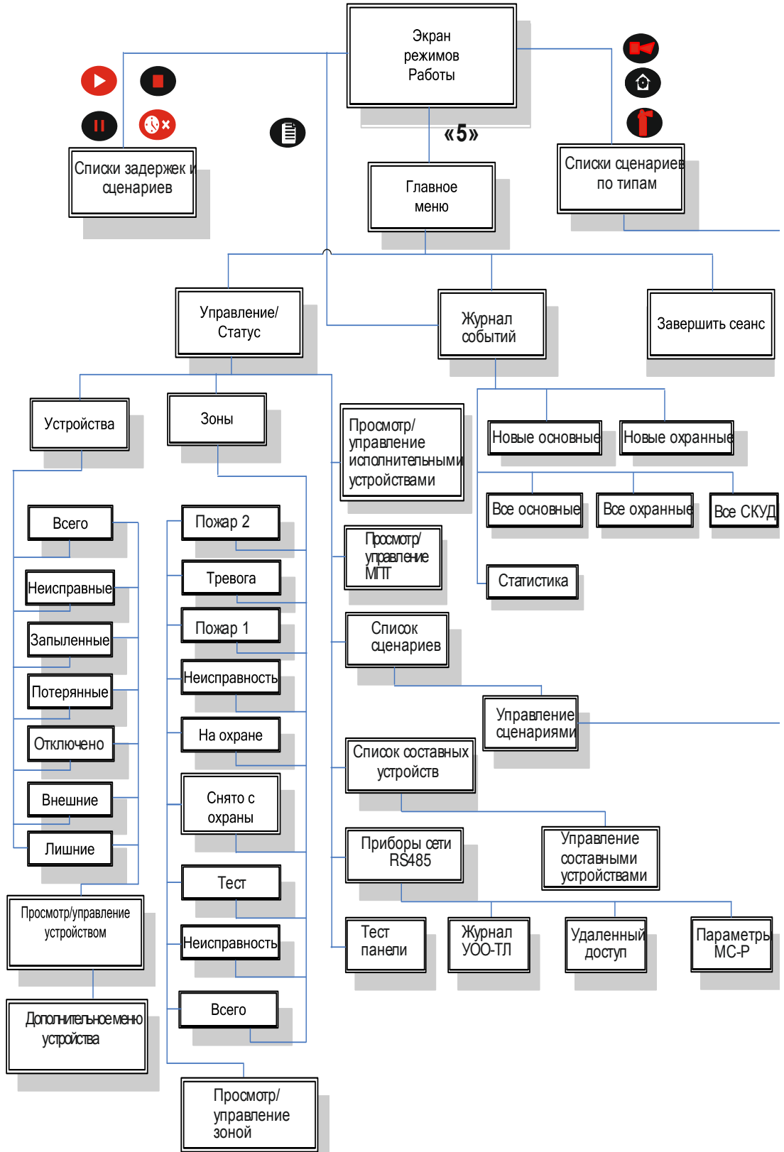
А.2 Структура экранов меню для уровня доступа «Дежурный» (окна, доступные первому уровню доступа показаны)
