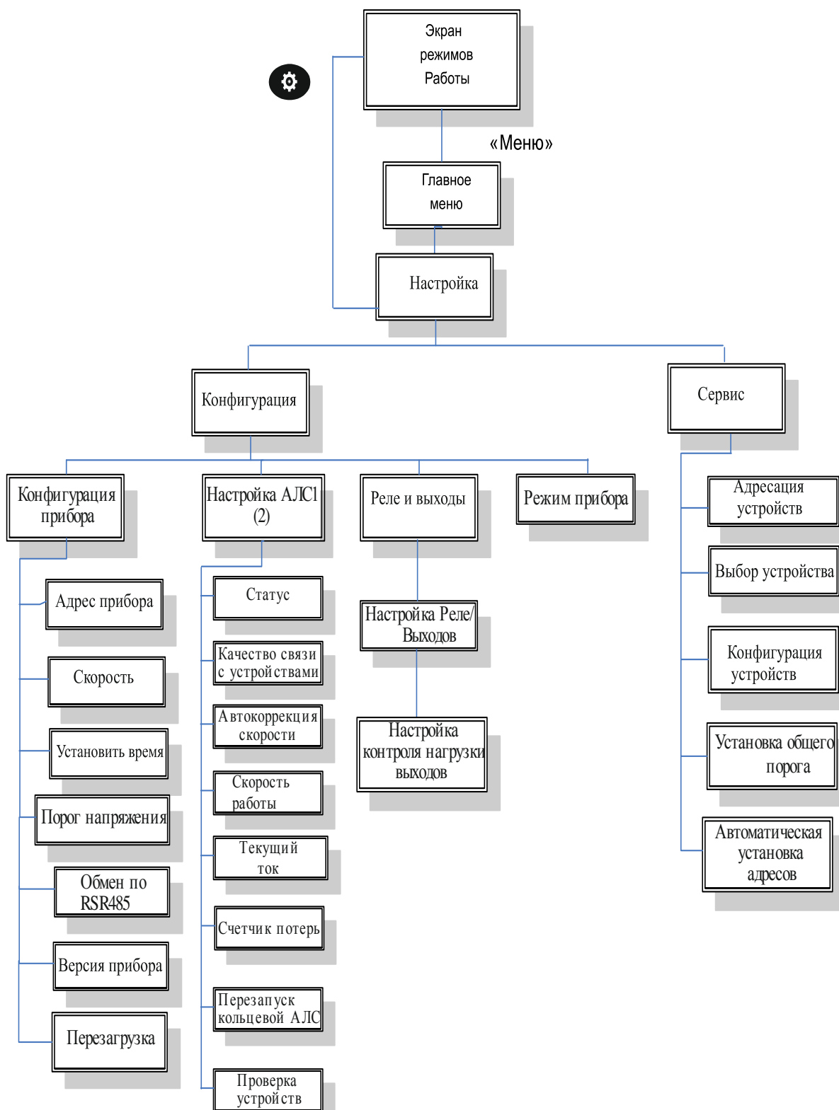
А.3 Структура экранов меню для уровня доступа «Инсталлятор» (окна, доступные первому и второму уровню доступа не показаны)
