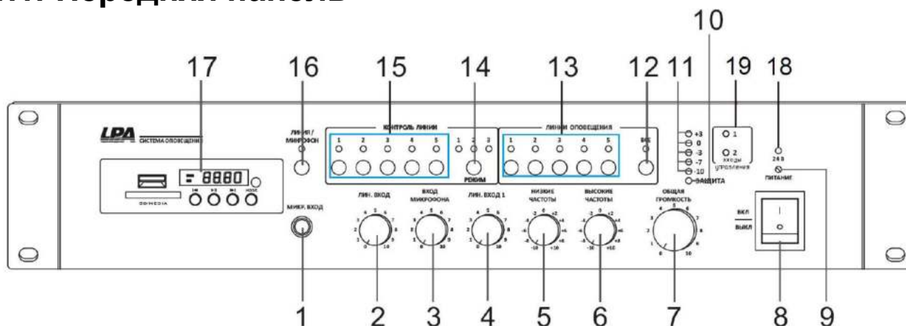
Рис. 1.2. Передняя панель
