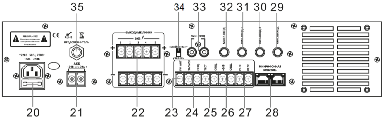
Рис. 1.3. Задняя панель
