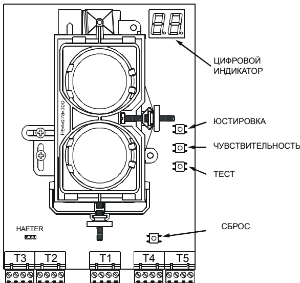
Рис. 6. Расположение кнопок
