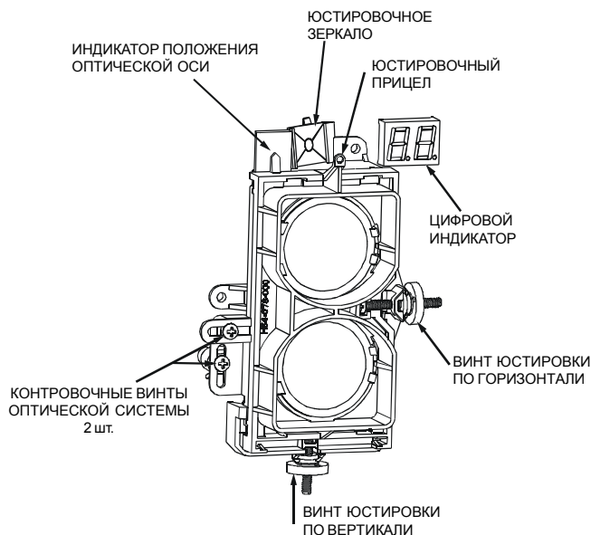
Рис. 7. Расположение органов юстировки
