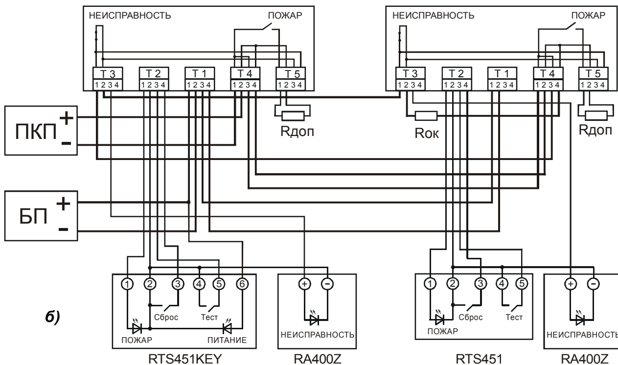
Рис. 5. Схемы подключения извещателей ИП212-125 (6500R) / ИП212-126 (6500RS) к ПКП:
