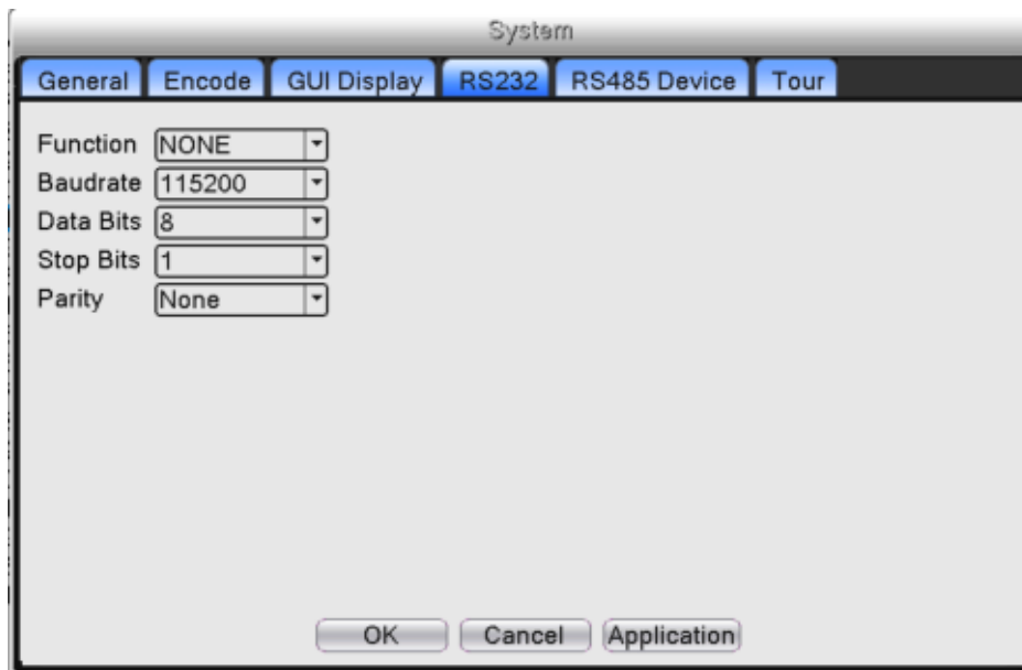
Рис.4.43 RS232
