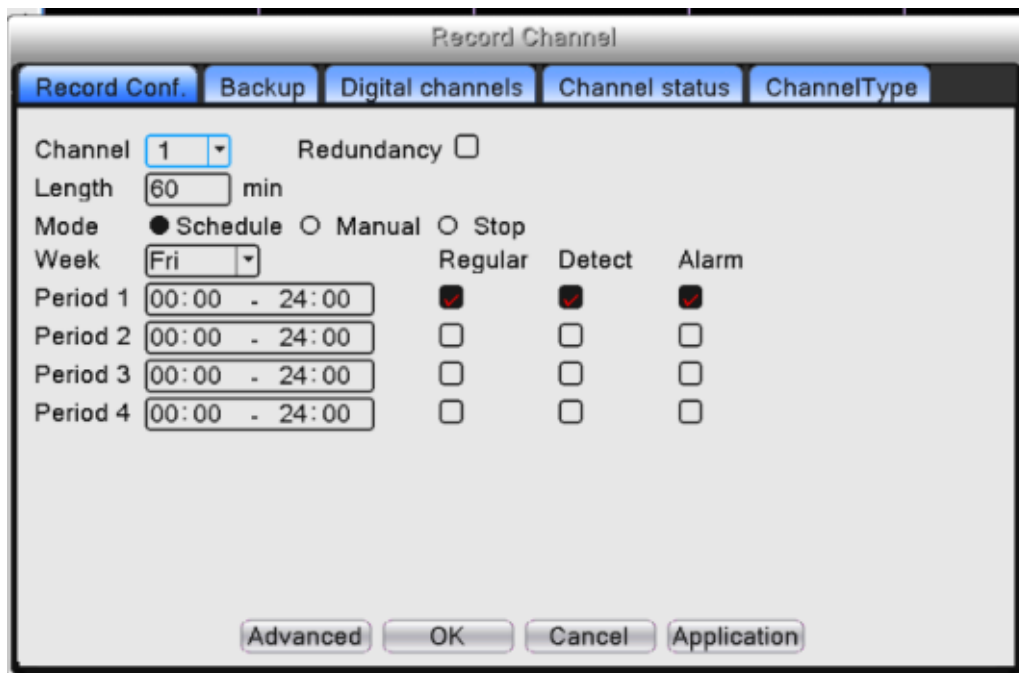
Рис.4.9 Настройка записи
