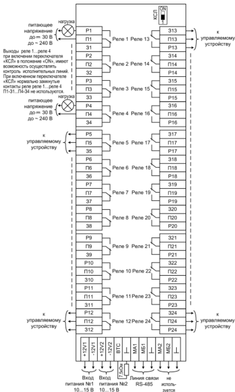
Рис.А7 Схема внешних подключений блока реле БР-24
