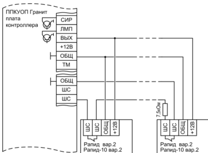
Рис.А4 Схема подключения охранных извещателей Рapid вар.2, Рapid-10 вар.2
