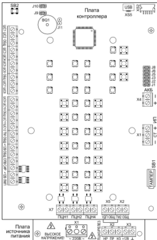
Рис.1 Плата контроллера Гранит-12А GSM (вид со снятой панелью индикации и управления) и плата источника питания (видимая часть)
