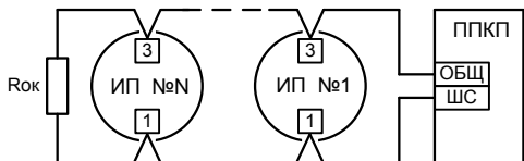
Рис.2 Типовая схема подключения извещателей
