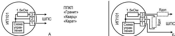
Рис.1 Схемы подключения извещателя к ШПС
