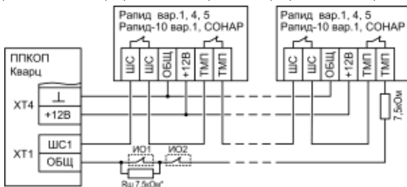
Рис.А9 Схема подключения охранных извещателей Репид вар.1,4,5, Репид-10 вар.1, СОНАР, ПОЛЮС-2 (ИО1, ИО2)
