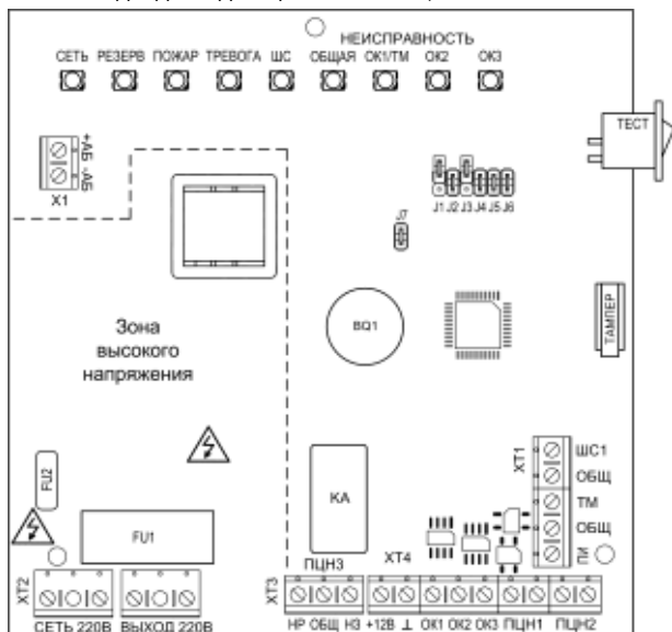
Рис.3 Плата прибора
