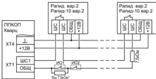
Рис.А8 Схема подключения охранных извещателей Репид вар.2, Репид-10 вар.2, ПОЛЮС-2 (ИО1, ИО2)
