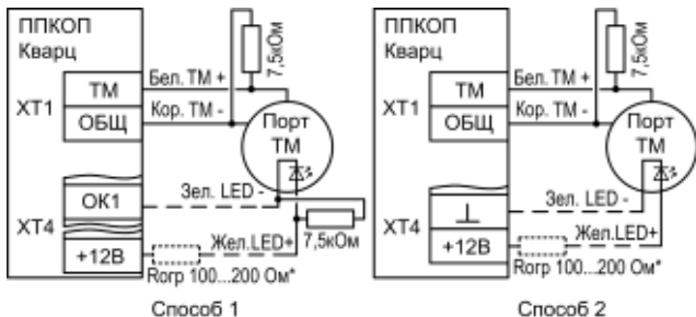
Рис.А2 Схемы подключения порта Touch Memory
