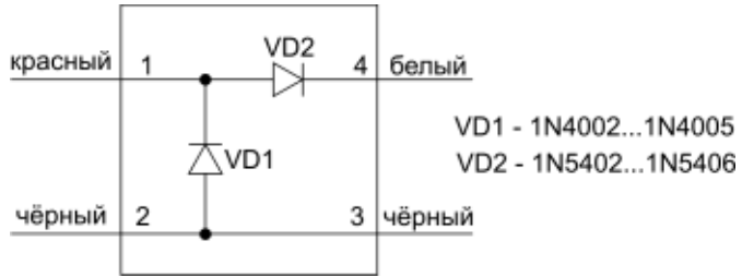
Рисунок 3. Схема модуля подключения нагрузки (МПН)
