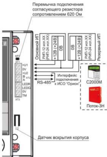
Рисунок 2. Схема внешних соединений блока «Поток-БКИ»
