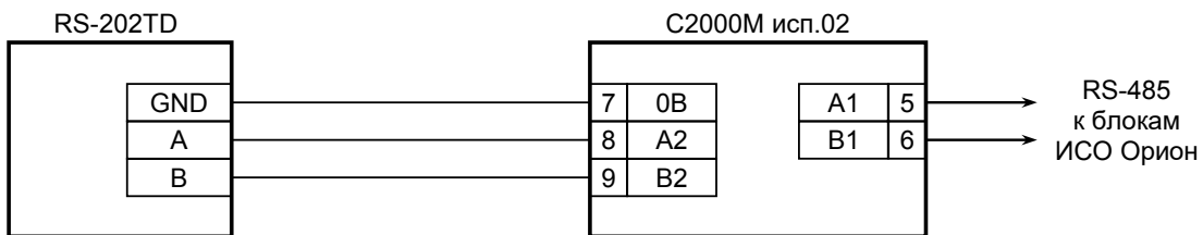
RS-202TD – радиопередатчик «Риф Стринг RS-202TD-RR»; C2000M исп.02 - пульт контроля и управления «C2000M исп.02».
