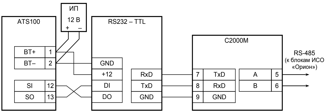
ATС100 – радиопередатчик ATС100; C2000M – пульт «C2000M»; RS232 – TTL – преобразователь RS232-TTL; ИП – резервированный источник питания
