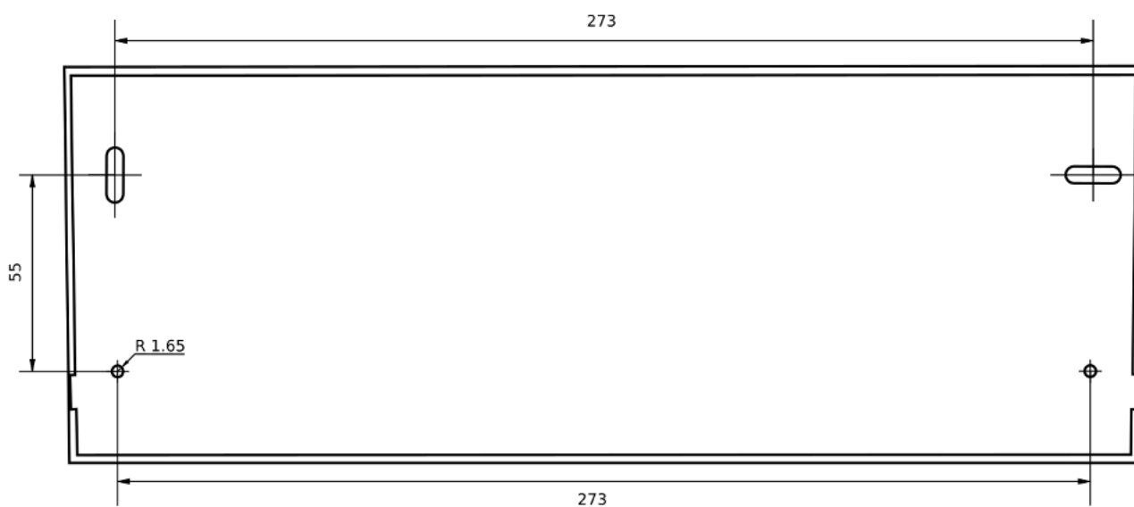
Рисунок 2.4 Монтажные размеры
