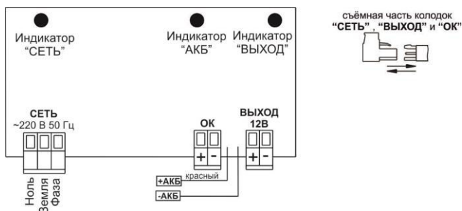
Рисунок 1 - вид изделия с открытой крышкой (схема подключения)
